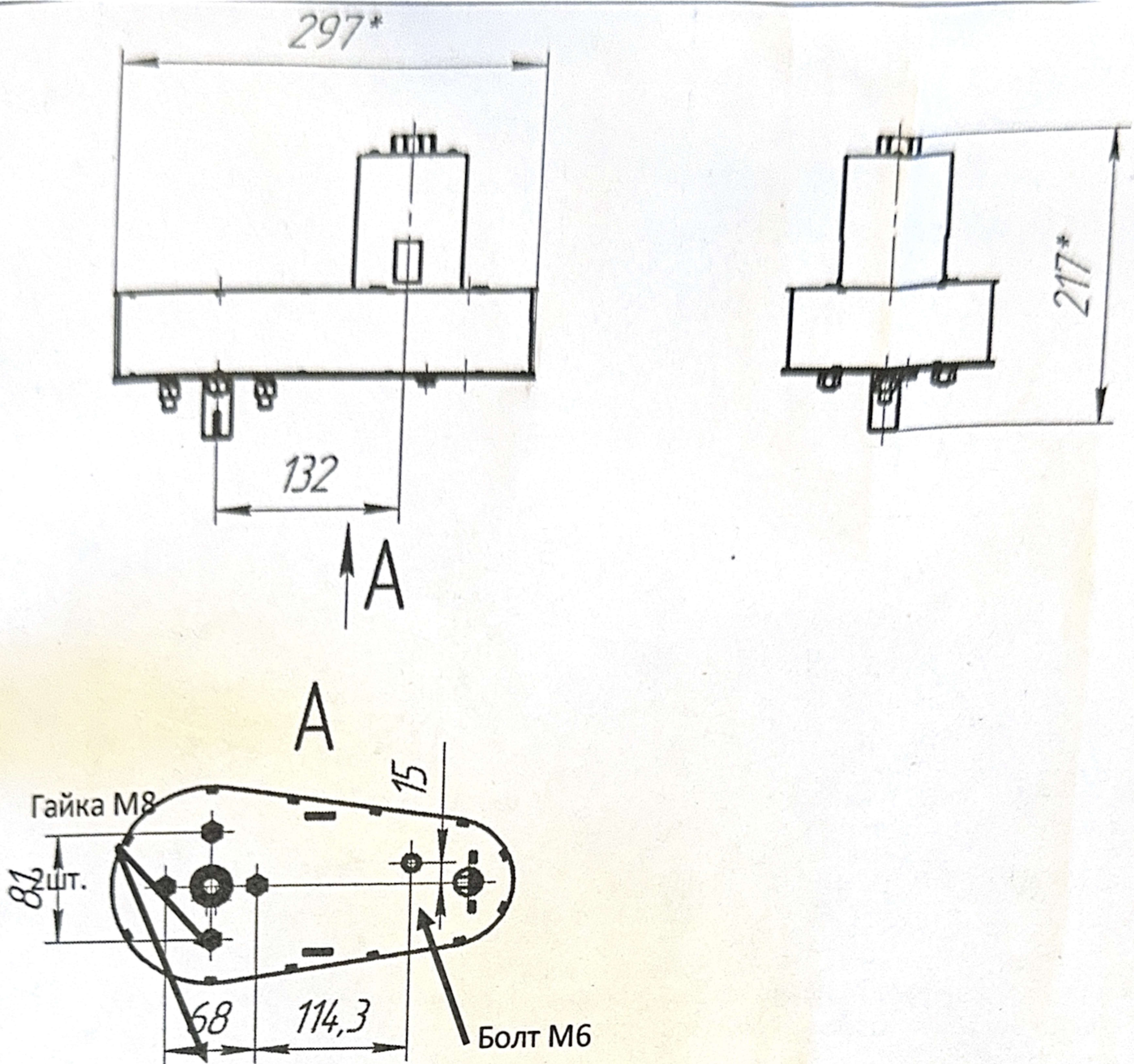
Рис. 1 Габаритные и установочные размеры редуктора.
