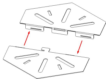
Рисунок 3. Сборка полки
