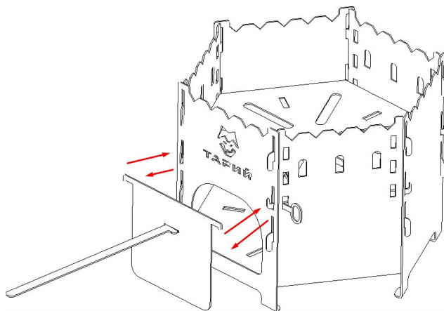
Рисунок 8. Снятие и установка дверки
