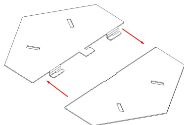
Рисунок 4. Сборка дна
