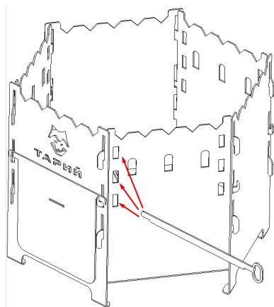
Рисунок 6. Места под спицу (крепёж полки)
