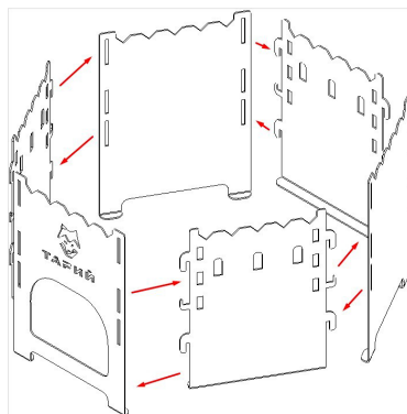
Рисунок 2. Сборка корпуса
